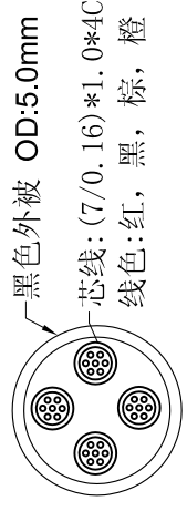
线规图
