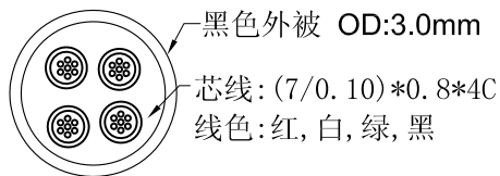
线规图
